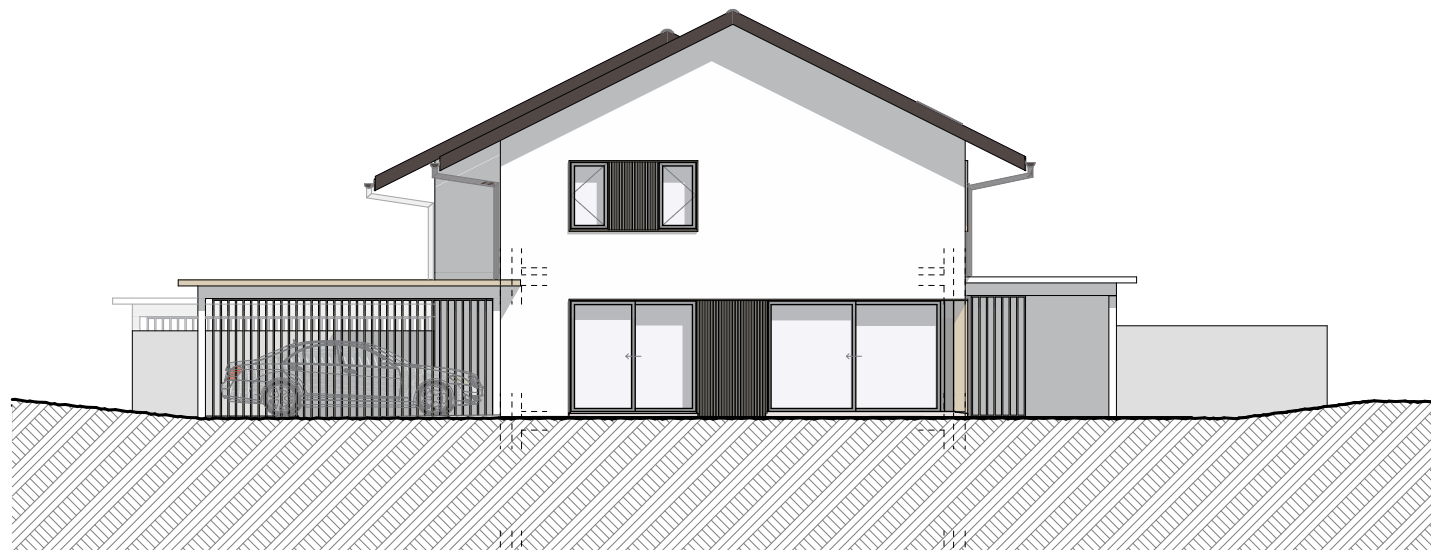
FACADE NORD-OUEST
